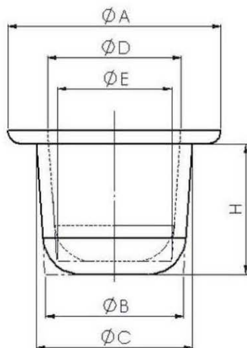
溝槽加工尺寸(單位：mm)
